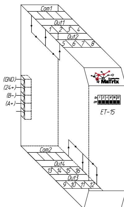
Рисунок 5 - Назначение контактов клемм
